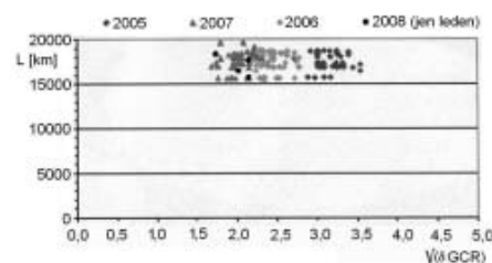
Obr. 3. Graf s údaji o spojeních stanice ZL3IX.
