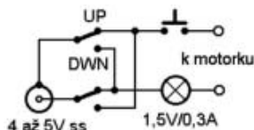
Obr. 6. Jednoduché zapojení obvodu napájení přeladovacího motorku.
