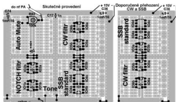
Obr.18. Pohled ze strany „mědi“ na základní umístění IO. IO jsou ze strany „izolantu“. Zkušební a zároveň definitivní destička plošného spoje 97x82 mm je ayy002 z Elektro-soud.cz Plzeň. Vpravo je doporučené přehození dílu CW a SSB – též na obr. 15a.
