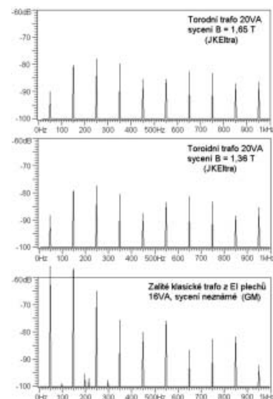
Obr. 12. Ukázky úrovní harmonických brumu ve vzdálenosti 5 cm pro toroidní trafo 20 VA JKEltra při sycení 1,65 T a 1,38 T a u klasického zatíženého trafo 16 VA (GM) při ss zatížení 2,5 W.
