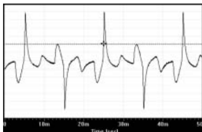
Obr. 13. Průběh primárního proudu popisovaného transformátoru 20 VA při zatížení zdroje ss proudem 100 mA. Naše zapojení z obr. 2 – 40 mA, klidový proud TDA2009 60 mA.
