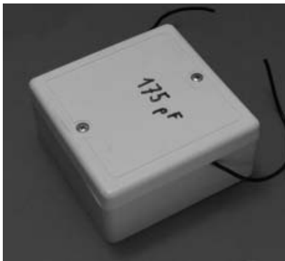
Obr. 5. Pevný VN kondenzátor pro ladící obvod vytvořený z koaxiálního kabelu RG58.
