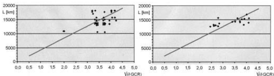
Obr. 2. Data o délkách spojení stanic VK6VZ (vlevo) a VK3ZL (vpravo), vynesena vůči \sqrt{\delta GCR} .
