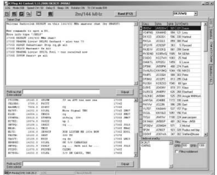
Obr. 5. Okno chat
