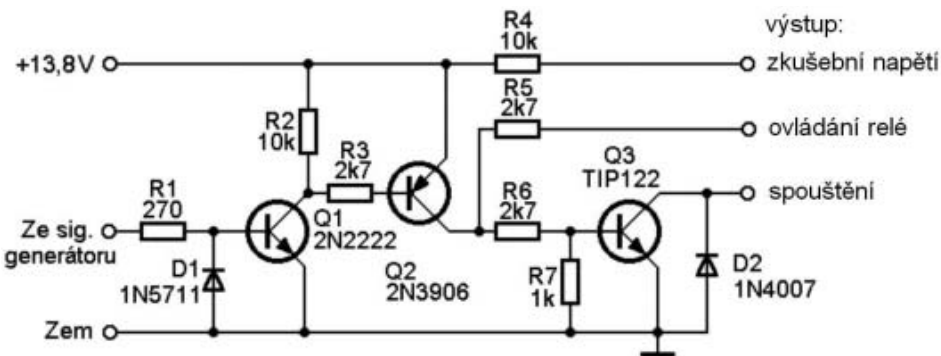
Obr. 5. Zapojení přípravku pro testování rychlosti spínání použitých relé. D1 1N5711, D2 1N4007, Q1 2N2222 (NPN), Q2 2N3906 (PNP), Q3 TIP122 – nebo jejich ekvivalenty. R1 270 Ω, R2, R4 10 kΩ, R3, R5, R6 2,7 kΩ, R7 1 kΩ. Všechny odpory 0,5 W.
