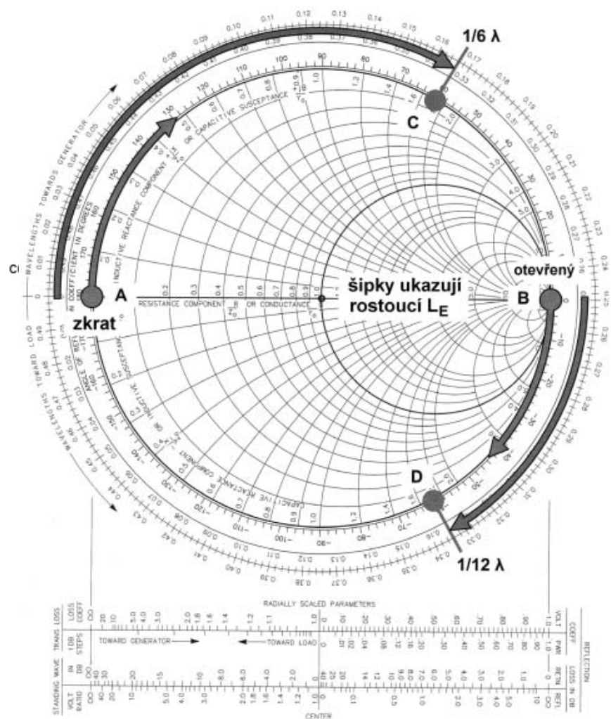
Obr. 4. Smithův diagram je vhodnou pomůckou pro popis chování vř vedení. Šipky z bodů A a B ukazují změny impedance zkratovaných a otevřených pahýlů s tím, jak roste jejich elektrická délka. Body C a D reprezentují impedance zkratovaného pahýlu \lambda/6 a otevřeného pahýlu \lambda/12 .
