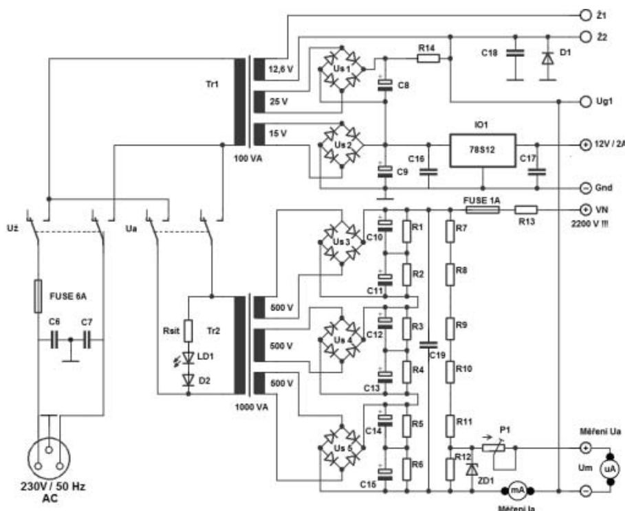
Obr. 3. Napájecí část
