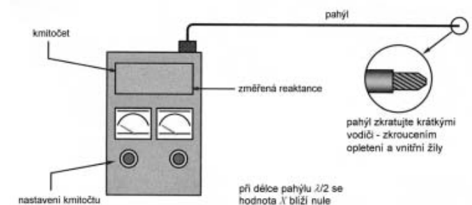
Obr. 2. Pro zkracování pahýlů na správnou elektrickou délku je vhodný SWR analyzátor (např. populární MFJ-259/269). Pro nejmenší kmitočet, při kterém se reaktance X blíží nule, je pahýl elektricky dlouhý \lambda/2 .
