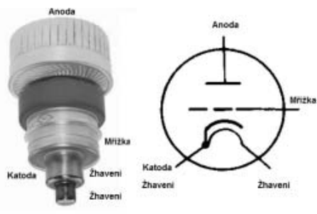
Obr. 2. Elektronka GI46b
