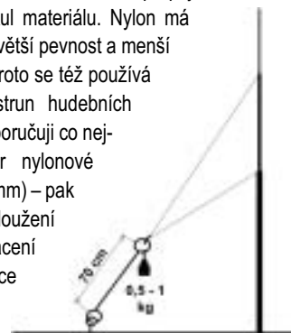
Obr. 3. Princip konstrukce kotvení vertikálu s pákami a závažími
