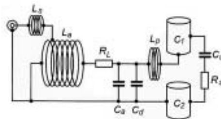
Obr. 7. Principální schéma EH antény
