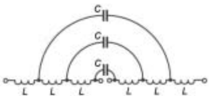
Obr. 2. Náhradní schéma dipólu
