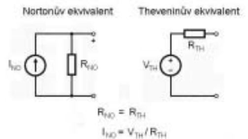
Obr. 3. Ekvivalentní Nortonův a Theveninův obvod vykazují na svých výstupech zcela shodné chování a jsou navzájem zaměnitelné.
