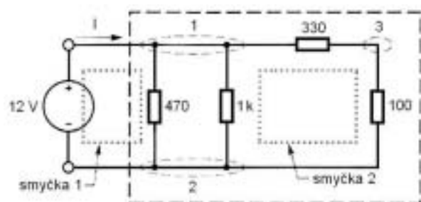
Obr. 3. Sestavte tento obvod a prověřte, jak rozumíte Kirchhoffovým zákonům.
