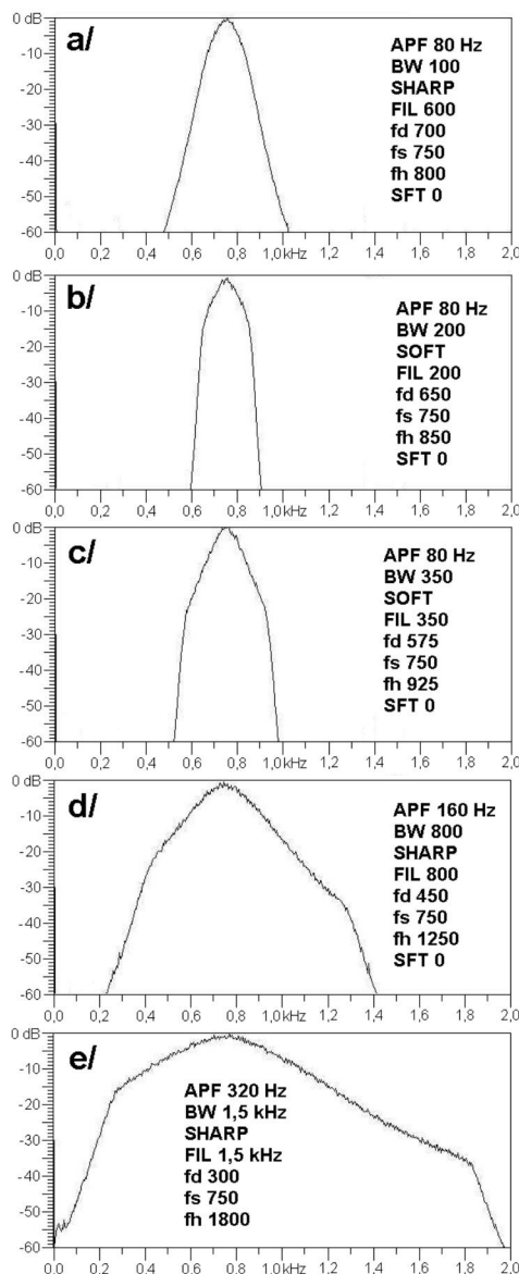
Obr. 4. Příklady nastavení praktických, účelných a dobře poslouchatelných křivek propustnosti pro CW. Výminkou je poslechově horší křivka b), které se ale někdy nevyhne.
