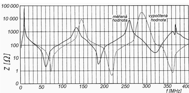
Obr. 7. Impedance koaxiální zadržky v kmitočtovém rozsahu od 1 do 400 MHz, je-li-li na koaxiální kabel pohlíženo jako na vedení
