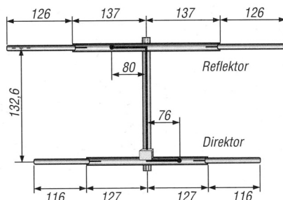
Obr. 2. Rozměrový náčrt antény HB9CV. Rozměry uváděny v cm.
