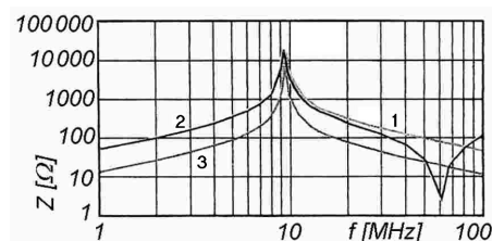
Obr. 4. Vypočtené hodnoty impedance v rozsahu 1-100 MHz pro obě náhradní schémata a naměřené hodnoty pro vzorek trapy z deseti závitů kabelu RG58. Křivka 1 - naměřené hodnoty, křivka 2 - vypočtené hodnoty pro 33,75 pF/8,4 mH, křivka 3 - vypočtené hodnoty pro 135 pF/2,1 mH.
