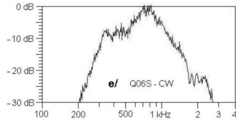
Obr. 6. Kmitočtová charakteristika reproboxů Genius SP-Q06S
