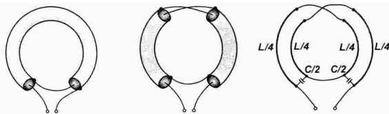
Obr. 1. Koaxiální zádrž sestávající z jednoho závitu, vnitřní vodič z konce závitu je spojen s opletením z jeho začátku. Obr. 2. Koaxiální zádrž, vnější vodič je přerušen a v místě rozdělení jsou vnitřní vodiče spojeny s protilehlými vnějšími vodiči. Obr. 3. Rozložení schématu z obr. 2 do čtyř oddělených indukčností a do dvou kapacit, které jsou vzhledem k přívodům zapojeny v sérii.
