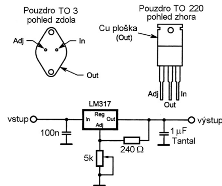
Obr. 3. Trisvorkový regulátor LM317 je velmi univerzální a odolný. Obvod je nutné doplnit vnějšími kondenzátory, aby vnitřní zesilovač regulátoru byly za všech podmínek stabilní. Odpor 240 Ω omezuje proud protékající potenciometrem 5 kΩ. Tento regulátor poskytuje nastavitelné výstupní napětí od cca 1,2 V až do maximální hodnoty, která je asi o 3 V menší, než je vstupní napětí.
