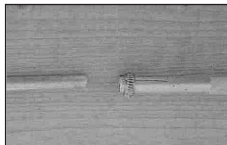
Obr. 5. Konce trubek 12 a 10 mm připravených k zasunutí a stažení hadicovou sponou
