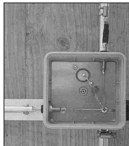
Obr. 4. Pohled na vnitřní uspořádání anténní přípojné krabice s konektorem PL a zdířkami
