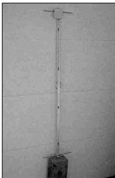
Obr. 1. Připravené ráhno s montážní krabicí, třmenem k upevnění ke stožáru a se závitovými tyčemi, které budou tvořit nosníky obou polovin zářiče i reflektoru.
