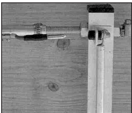
Obr. 7. Ukázka spoje mezi částmi fázovacího vedení nad reflektorem a nad ráhmem
