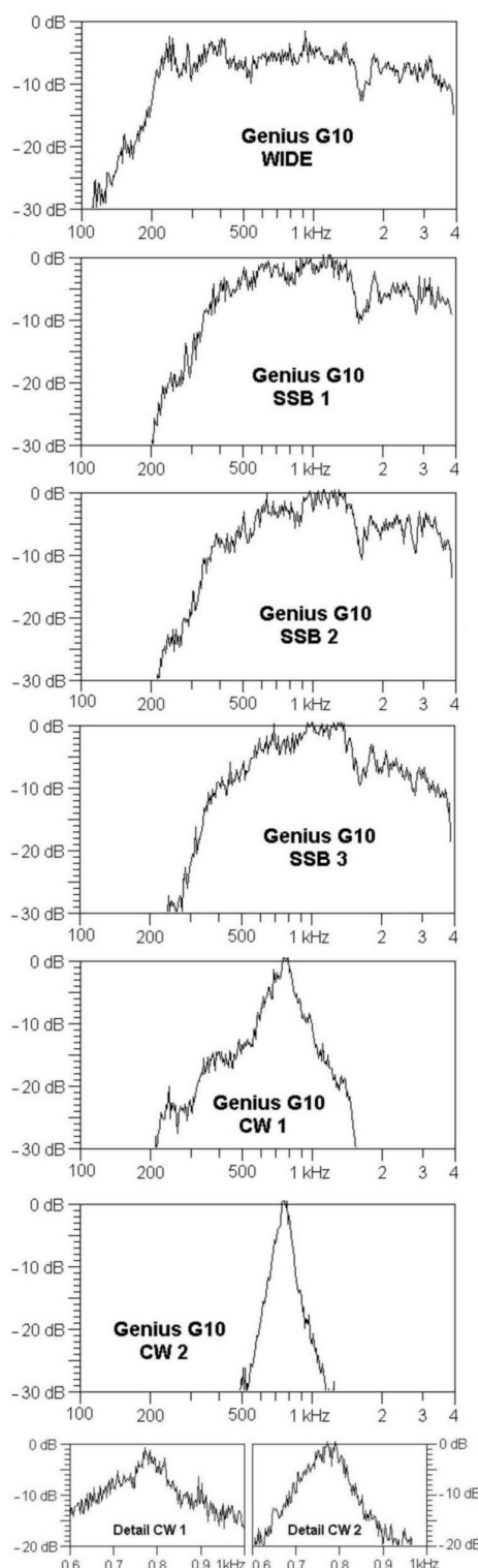
Obr. 9. Kmitočtové charakteristiky boxů G10
