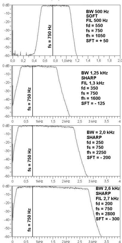
Obr. 2. Kontrola nastavení námi zvolených středů CW filtrů 750 Hz
