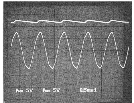
Obr. 3. Obrázek ukazuje průběh sinusového vstupního napětí a výstupního napětí na kondenzátoru C2 u půlvlnného zdvojovače. Všimněte si, že kondenzátor C2 se nabíjí vždy jednou během každé druhé půlvlny. Nulová hodnota potenciálu je pro oba průběhy umístěna ve středu (v ose) sinusové vlny.
