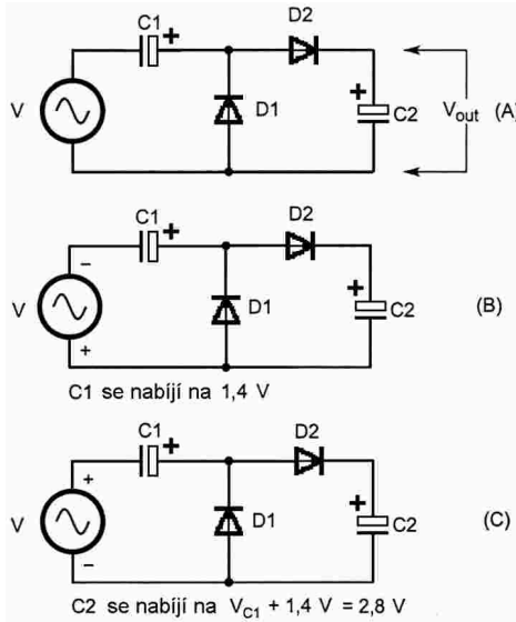
Obr. 1. Půlvlnný zdvojovač napětí. Obr. 1 B a 1 C ukazují, jak se jednotlivé kondenzátory nabíjejí během následujících půlvln. Napětí na kondenzátorech C1 a C2 se sečítají.
