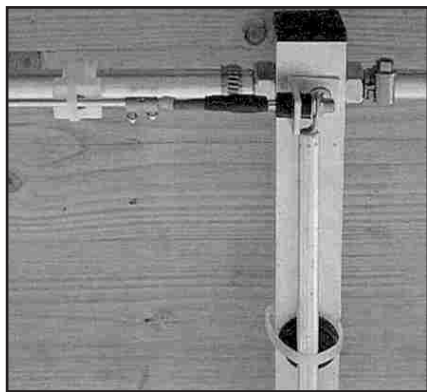
Obr. 6. Izolovaná upevněná zdířka na ráhnu s připojenou šestimilimetrovou trubicí fázovacího vedení
