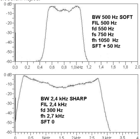
Obr. 7. Pokazení kmitočtových charakteristik funkcí NR v poloze 11 hodin, porovnejte s obr. 1b a obr. 5.
