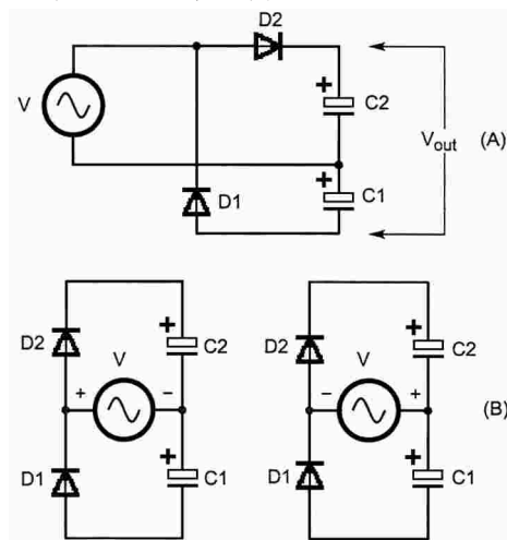
Obr. 2. Celovlnný, dvojčinný zdvojovač napětí. Schéma nakreslené běžným způsobem je na obr. 2 A, názorněji překreslené schéma, které také ilustruje, jak jsou během jednotlivých půlvln nabíjeny kondenzátory, je na obr. 2 B.
