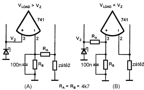
Obr. 2 A. Napěťový dělič z odporů RA a RB způsobí, že operační zesilovač bude řídit sériový regulační tranzistor tak, že napětí na zátěži bude větší, než napětí na Zenerově diodě. B. Stejný nápad použijeme pro napětí na zátěži menší, než napětí Zenerovy diody.
