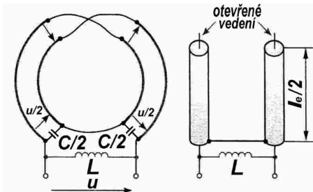
Obr. 5. Náhrada indukčnosti vedení soustředěnou indukčností L , zapojenou na svorkách zadržky (vlevo). Obr. 6. Náhradní schéma vedení po přerušení v místě, kterým neprochází žádný proud.
