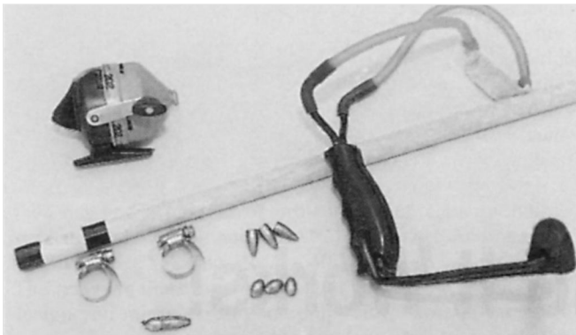
Obr. 1. Vrhací antény. Skládá se z praku, levného rybářského navijáku a dřevěné tyčky. Naviják uchytkuje k tyčce hadicovými sponami. Dráhu letu ovlivňuje volbou vhodného rybářského závažíčka.
